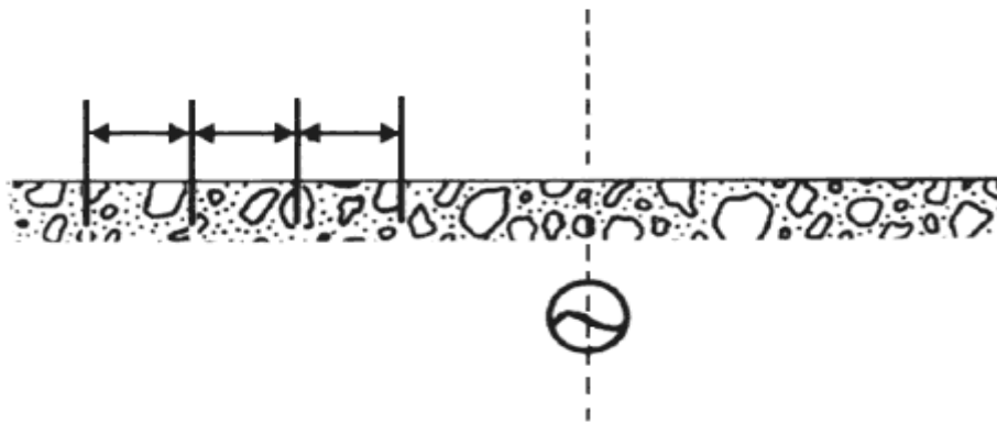
Figura 2. Disposición correcta de los cuatro electrodos.
